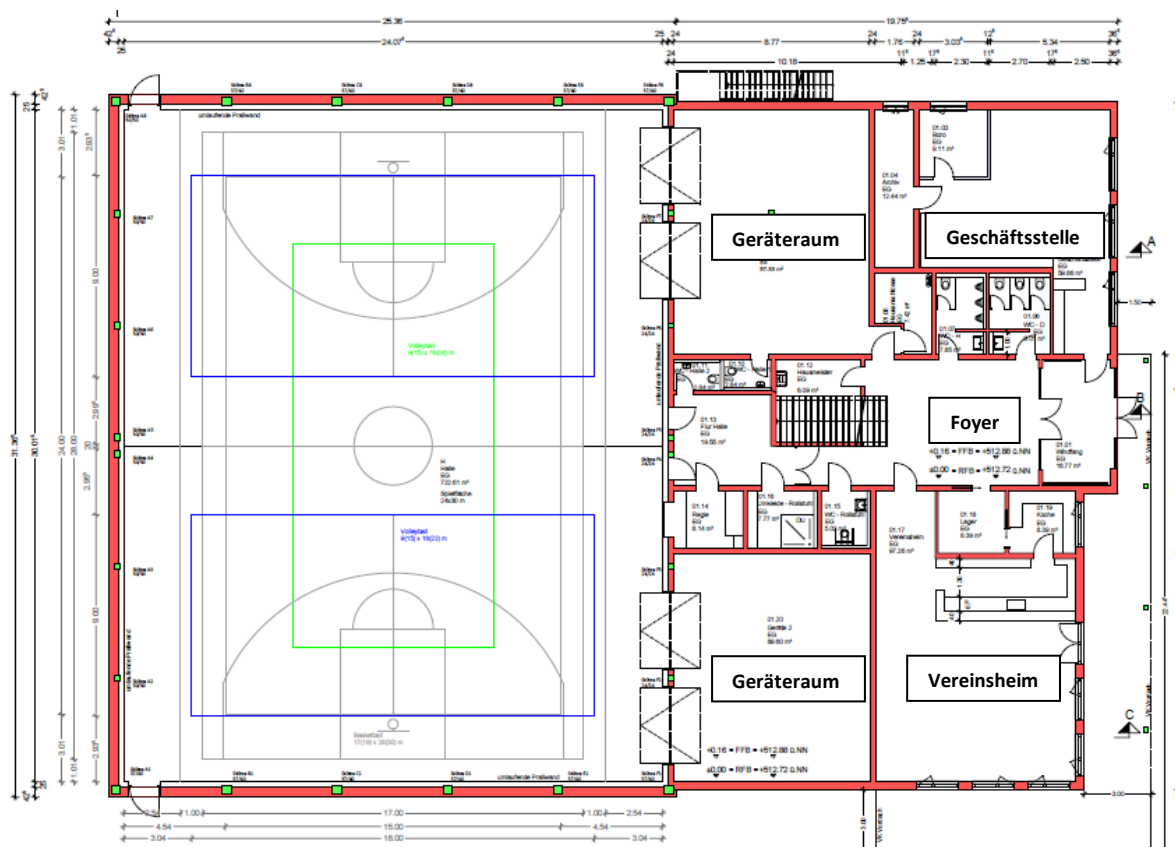
Bruckhofstraße, Grundriss der Halle
